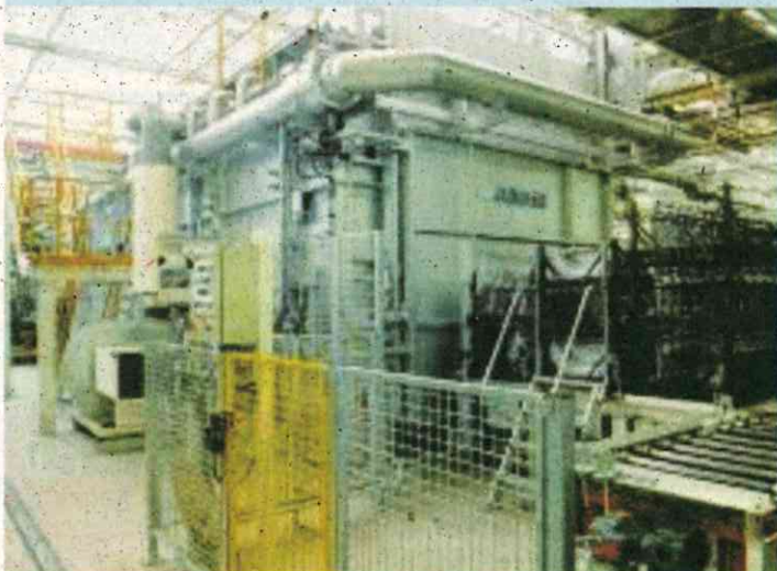
Pec na tepelné zpracování hliníkových dílů.
